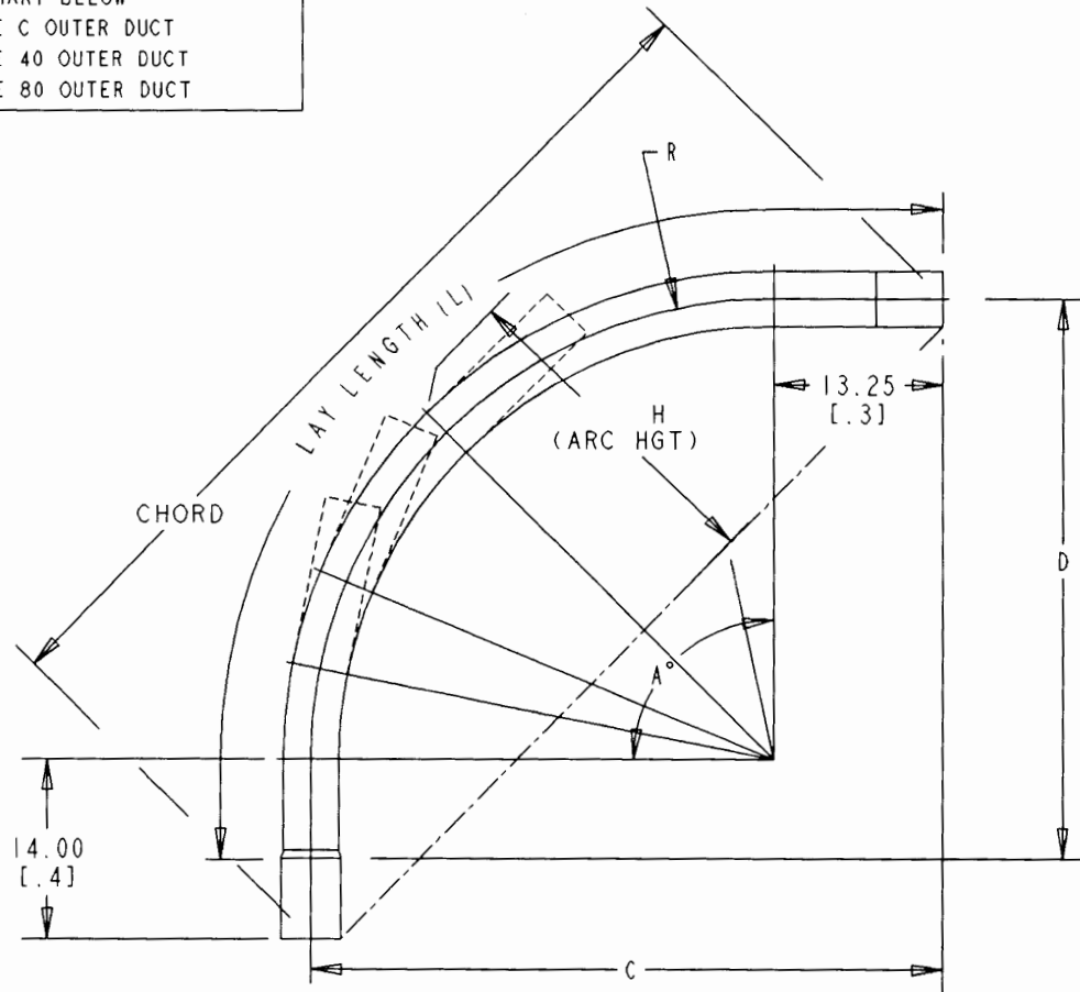
DIMENSIONS - INCHES (METERS)
